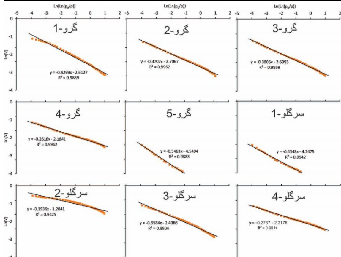
شکل ۳: نمودار LnV در مقابل Ln(Ln(P/P)) نمونه های مطالعه شده جهت اندازه گیری میزان بعد فرکتال
