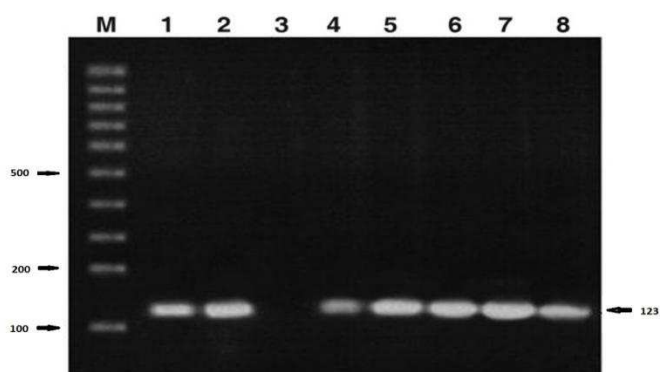
شکل ۱. الگوی حاصل از تکثیر PCR-RFLP
