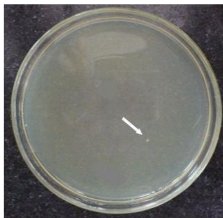
شکل ۳- نتایج ترانسفورماسیون باکتری E. coli XL1-Blue با وکتور نو ترکیب حاوی ژن اینترفرون بتا
