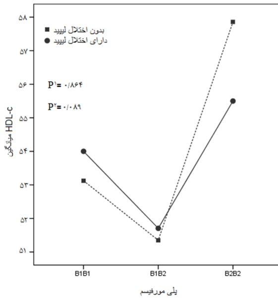
شکل ۱- مقایسه میانگین لگاریتم HDL-C در سه ژنوتیپ مربوط به پلی مورفیسم CETP Taq1B دو گروه دارای اختلال لیپید ( TG \geq 150 \text{mg/dl} و TC \geq 200 \text{mg/dl} ) و بدون اختلال لیپید ( TG < 150 \text{mg/dl} و TC < 200 \text{mg/dl} )
