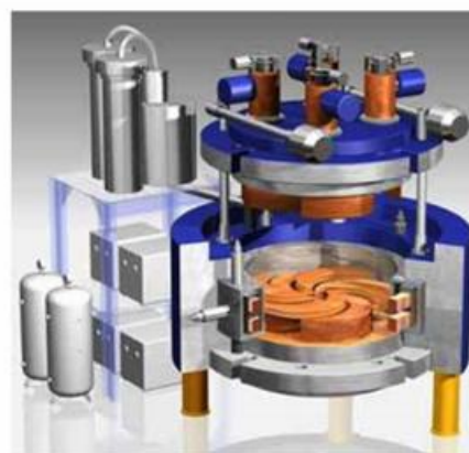
شکل ۶- مسیر ذرات در یک سیکلوترون که همزمان در یک میدان الکتریکی و مغناطیسی شتاب می‌گیرند (چپ). نمایی از یک سیکلوترون با استفاده از ابرسانها که منجر به کاهش وزن آن تا ۸۰ تن گردیده است. ساخت کمپانی آلمانی ACCEL (راست).
