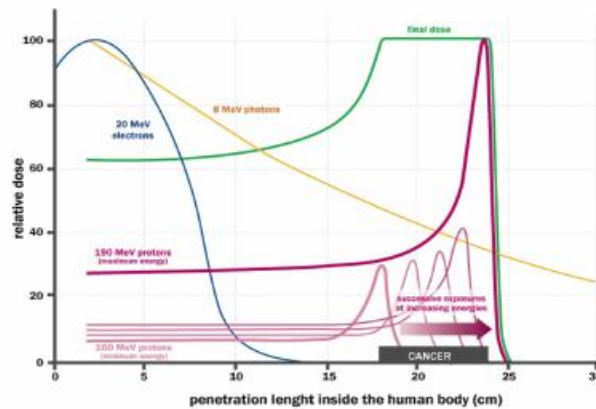
شکل ۲- نمودار توزیع دز نسبی بر حسب عمق نفوذ در بافت های بدن برای نظیر الکترون، فوتون و پروتون. بر طبق نمودار، الکترون و فوتون بخش اعظم انرژی را را لایه های سطحی آزاد می کنند در حالی که پروتون قابلیت تحویل دز را در لایه های عمقی تر (تومور) و قابلیت تنظیم برد با تغییر انرژی را دارد و در نتیجه باعث حفظ بیشتر بافت های سالم نظیر آنچه در شکل ۳ نشان داده شده نیز می گردد (۱۵).
