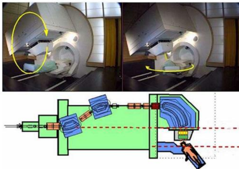
شکل ۱۲- گانتري مرکز پروتون درمانی PSI، سوئیس
