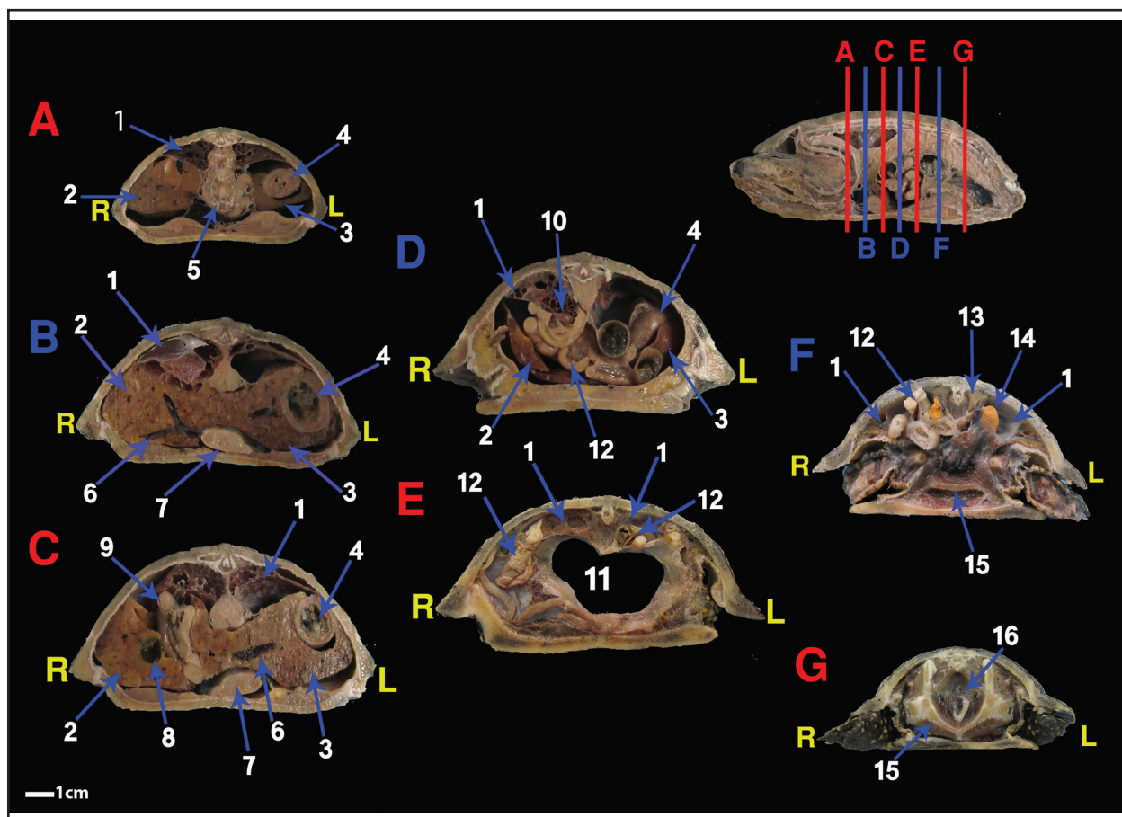
تصویر ۲. بررسی کالبدشناسی برش عرضی حفره سلومی، لاک‌پشت برکه‌ای اروپایی. ۱. Lung، ۲. Left lobe of the liver، ۳. Right lobe of the liver، ۴. Stomach، ۵. Neck، ۶. Cloaca، ۷. Vessels of the liver، ۸. Heart، ۹. Gall bladder، ۱۰. Duodenum، ۱۱. Spleen، ۱۲. Urinary bladder، ۱۳. Intestine، ۱۴. Kidney، ۱۵. Testis، ۱۶. Pelvic girdle.
