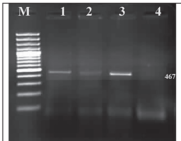
تصویر ۲. تصویر ژل آگارز: ردیابی ژن gyrA یرسینیا راکری با تکنیک PCR. لاین M: مارکر ۱۰۰ جفت بازی، لاین‌های ۱، ۲ و ۳: نمونه‌های مثبت ژن gyrA ، لاین ۴: کنترل منفی.
