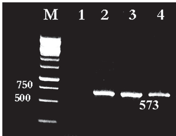
تصویر ۱. تصویر ژل آگارز: ردیابی ژن ۱۶SrRNA یرسینیا راکری با تکنیک PCR. لاین M: مارکر ۱۰۰ جفت بازی، لاین ۱: کنترل منفی، لاین ۲ و ۳: نمونه‌های مثبت یرسینیا راکری، باند ۴: کنترل مثبت.
