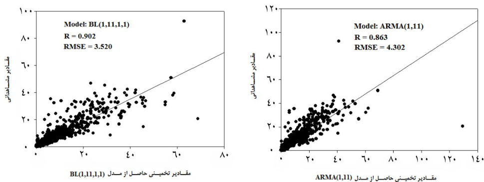
شکل ۲- نمودار پراکندگی مقادیر مشاهده‌ای و تخمینی به‌دست آمده از مدل‌های خطی و غیرخطی برای سری روزانه رودخانه باراندوزچای در مرحله صحت‌سنجی (۸۸-۱۳۸۴).
