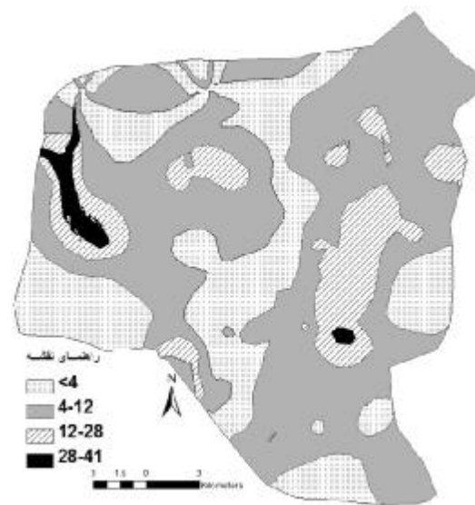
شکل 8- نقشه هدایت هیدرولیکی (m day -1 ).
