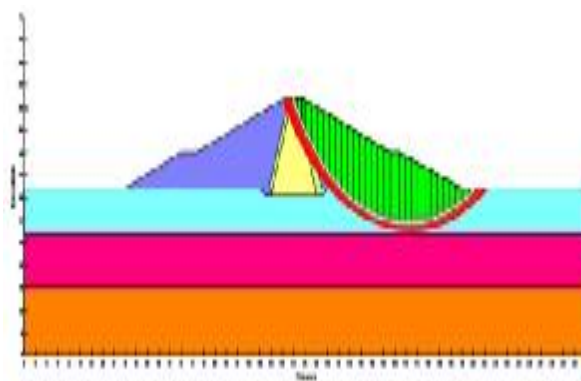
شکل 9- سطح لغزش برای شیب پایین دست بعد از پایان عملیات ساخت.
