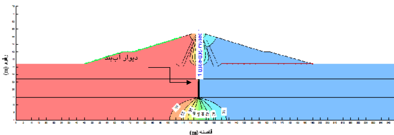
شکل 6- دبی عبوری از مقطع عمیق و خطوط همپتانسیل برای حالت با دیوار آب‌بند.
