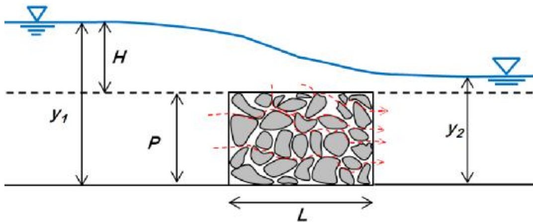
شکل 1- نمایی از مدل فیزیکی استفاده شده در آزمایش و پارامترهای آن.
