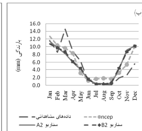
شکل 2- مقایسه بارش ماهانه مشاهده‌ای و شبیه سازی شده توسط مدل در دو دوره واسنجی (الف) و صحت سنجی (ب) ایستگاه بم
