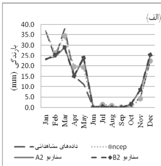
شکل 1- مقایسه بارش ماهانه مشاهده‌ای و شبیه سازی شده توسط مدل در دو دوره واسنجی (الف) و صحت سنجی (ب) ایستگاه کرمان
