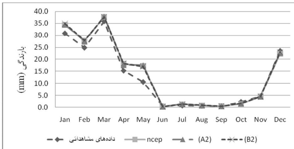
شکل 3- مقایسه بارش ماهانه مشاهده‌ای و شبیه‌سازی شده توسط مدل دوره پایه ایستگاه کرمان
