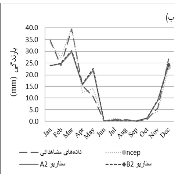
شکل 1- مقایسه بارش ماهانه مشاهده‌ای و شبیه سازی شده توسط مدل در دو دوره واسنجی (الف) و صحت سنجی (ب) ایستگاه کرمان
