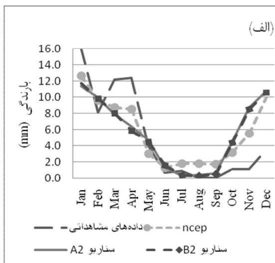
شکل 2- مقایسه بارش ماهانه مشاهده‌ای و شبیه سازی شده توسط مدل در دو دوره واسنجی (الف) و صحت سنجی (ب) ایستگاه بم
