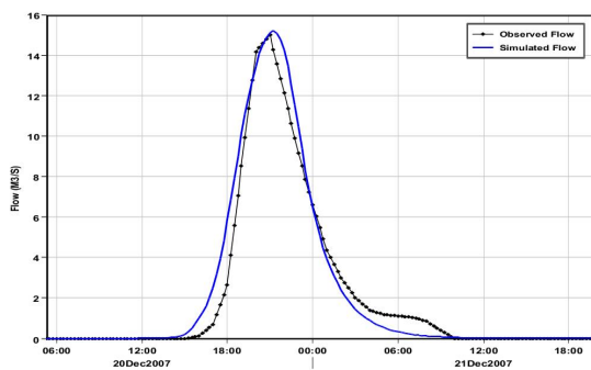
شکل 5 - هیدروگراف مشاهده‌ای و شبیه‌سازی پس از واسنجی برای رویداد 20 دسامبر 2007
