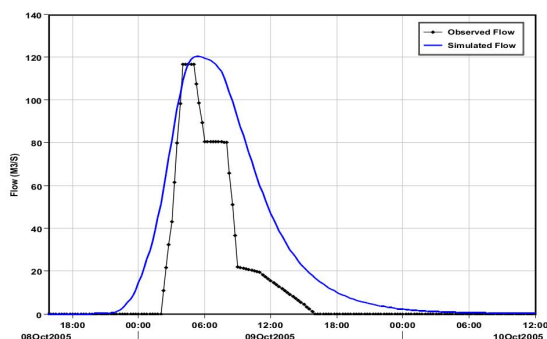
شکل 11- هیدروگراف مشاهده‌ای و شبیه‌سازی در مرحله اعتبارسنجی برای رویداد 9 اکتبر 2005
