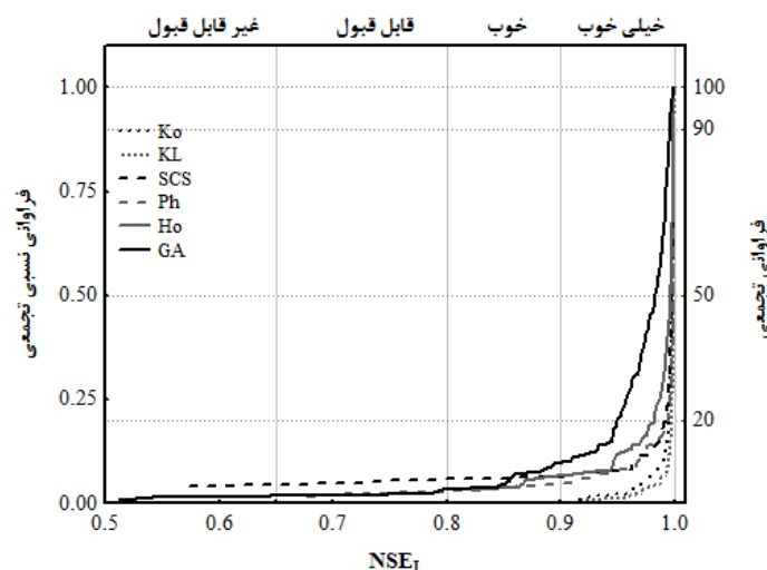
شکل ۳- توزیع تجمعی آماره NSE_I برای مدل‌های نفوذ آب به خاک Figure 3- cumulative distribution of NSE_I index for Soil Water Infiltration Models
