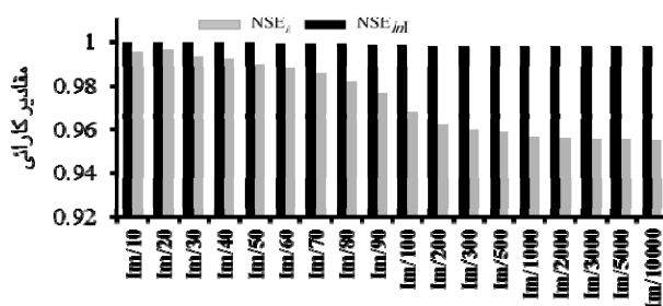
شکل ۵- تغییرات مقادیر میانگین NSE_{II} و NSE_{Iml} برای مدل کوستیاکف در یک خاک برای مقادیر مختلف \epsilon (Im میانگین نفوذ تجمعی (سانتی‌متر))
