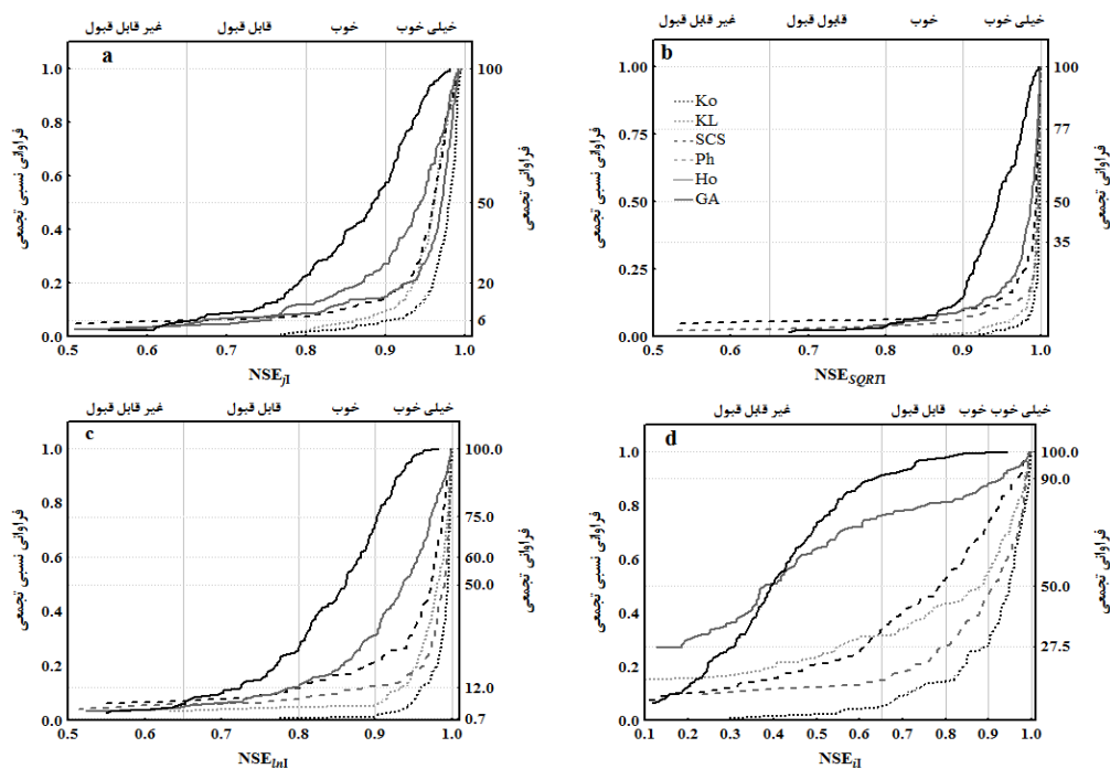
شکل ۴- توزیع تجمعی آماره‌های (a) NSE_{II} , (b) NSE_{SQRTI} , (c) NSE_{Iml} , (d) NSE_{II} برای مدل‌های نفوذ آب به خاک
