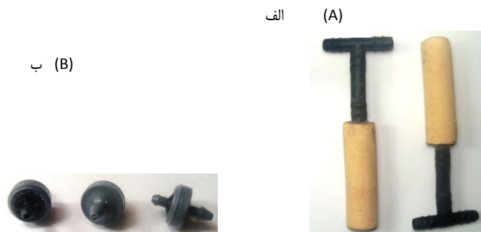
شکل ۱- نازل‌های بکار رفته در آبیاری زیرسطحی (الف) و سطحی (ب). الف، کپسول رسی متخلخل G 15 و ب، قطره چکان نتافیلیم چهار لیتر بر ساعت می‌باشد.
