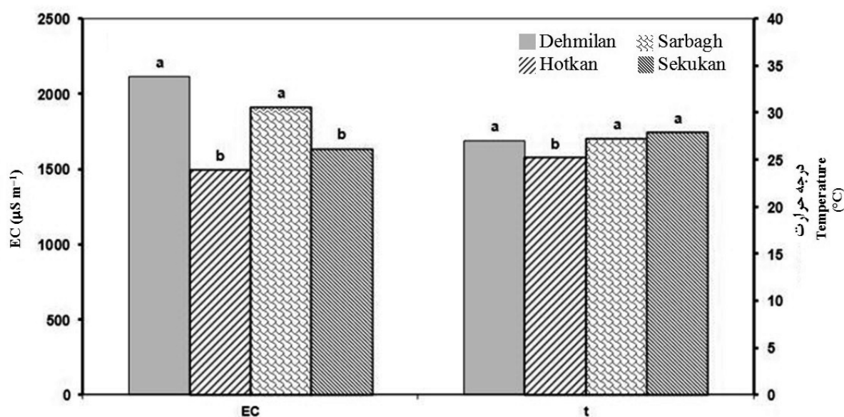
شکل ۳- مقایسه هدایت الکتریکی و درجه حرارت اندازه‌گیری شده در خروجی سیستم‌های تصفیه مورد مطالعه
