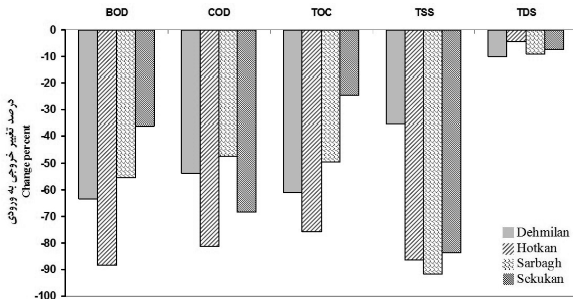
شکل ۶- مقایسه درصد تغییر خروجی نسبت به ورودی برای برخی خصوصیات در سیستم‌های تصفیه Figure 6- Comparison of change percent of wastewater properties at the outlet ratio to the inlet values in the refining systems
