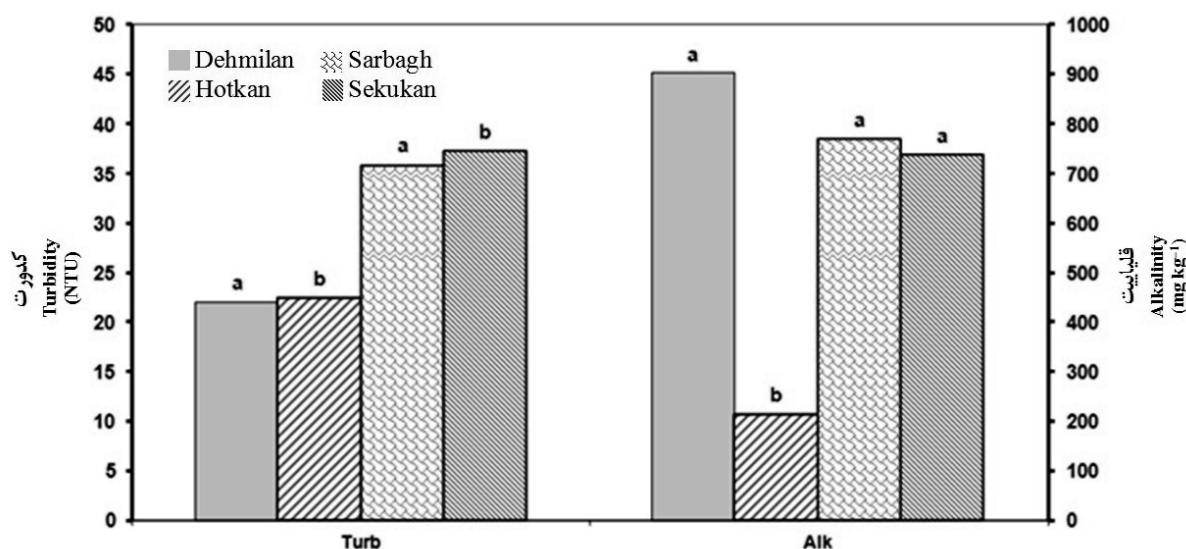
شکل ۴- مقایسه کدورت و قلیائیت اندازه‌گیری شده در خروجی سیستم‌های تصفیه مورد مطالعه
