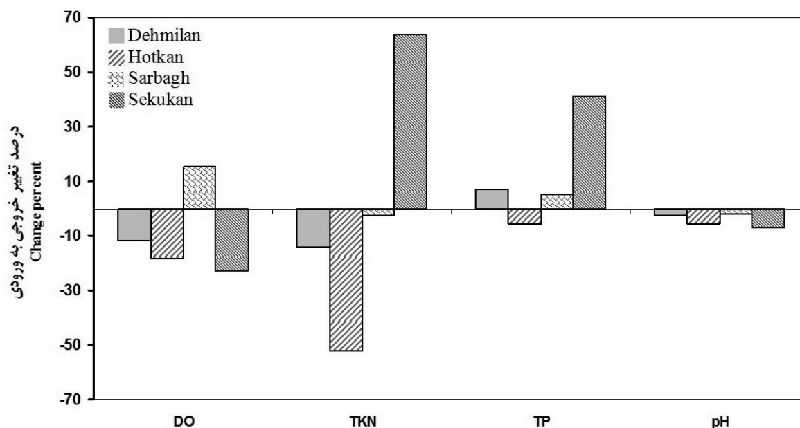
شکل ۷- مقایسه درصد تغییر خروجی نسبت به ورودی برای برخی خصوصیات در سیستم‌های تصفیه
