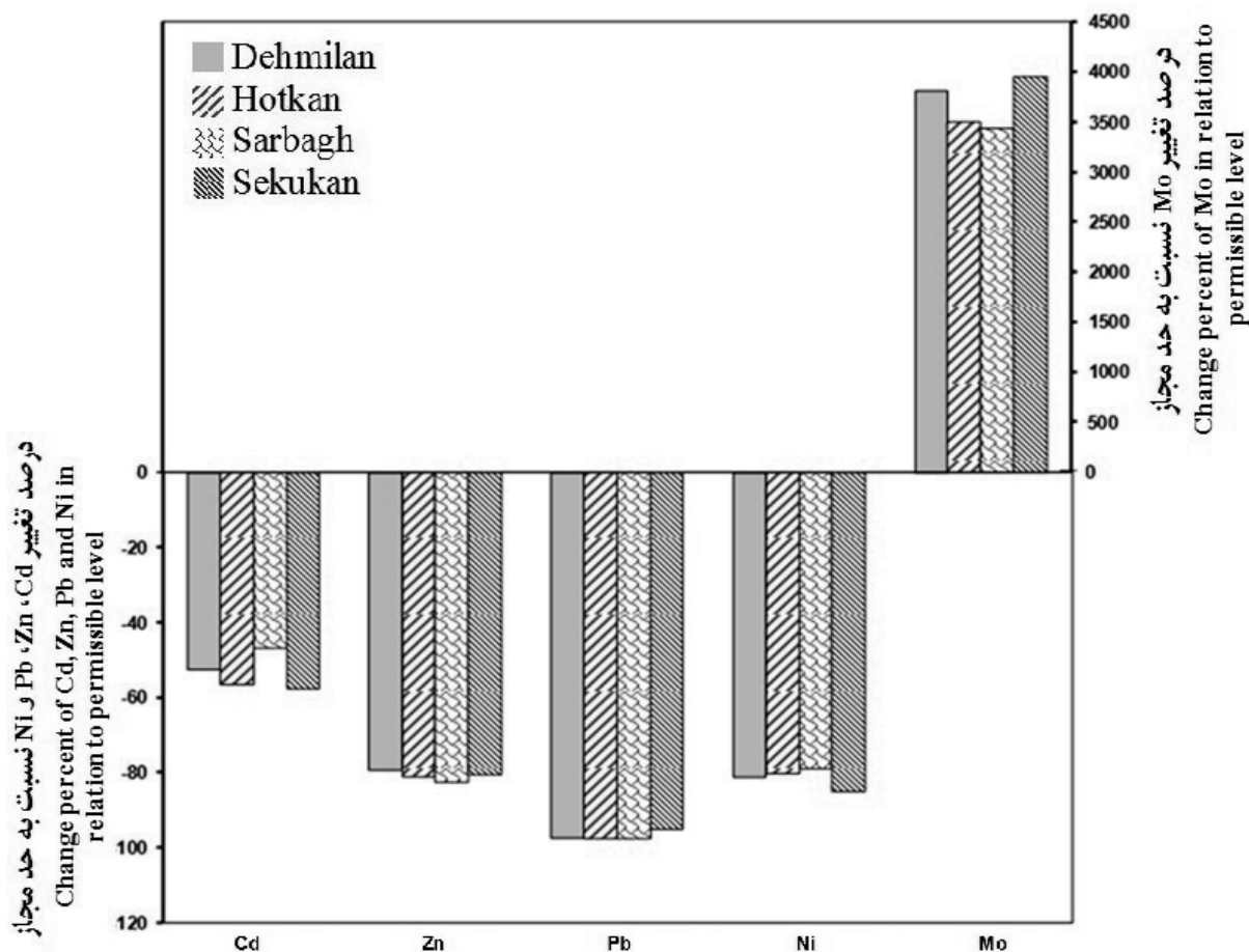
شکل ۱۱- مقایسه درصد تغییر غلظت عناصر سنگین در خروجی نسبت به حد مجاز در سیستم‌های تصفیه
