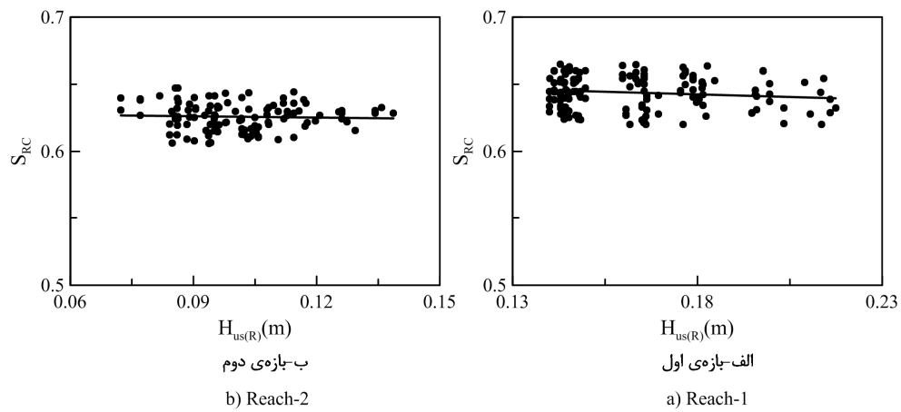
شکل 10- تأثیر عمق اولیه‌ی آب بر روی شاخص حساسیت انتقال بازه Figure 10- Effect of initial water depth on conveyance index
