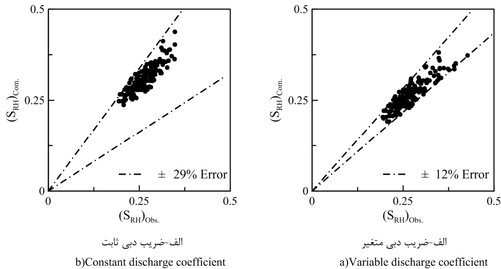
شکل 7- شاخص حساسیت S_{RH} مشاهده‌ای و محاسبه‌ای برای بازه‌های مجموعه‌ای آزمایشگاهی Figure 7- Observed and calculated values of reach sensitivity indicator of water depth
