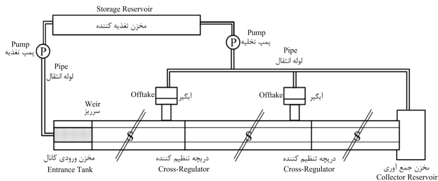
شکل 1- نمایی کلی از مجموعه‌ی آزمایشگاهی Figure 1- Schematic of the experimental setup plan
