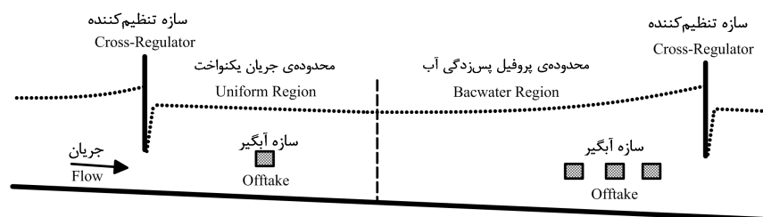
شکل 2- وضعیت کنترل جریان در یک بازه از شبکه‌ی آبیاری
