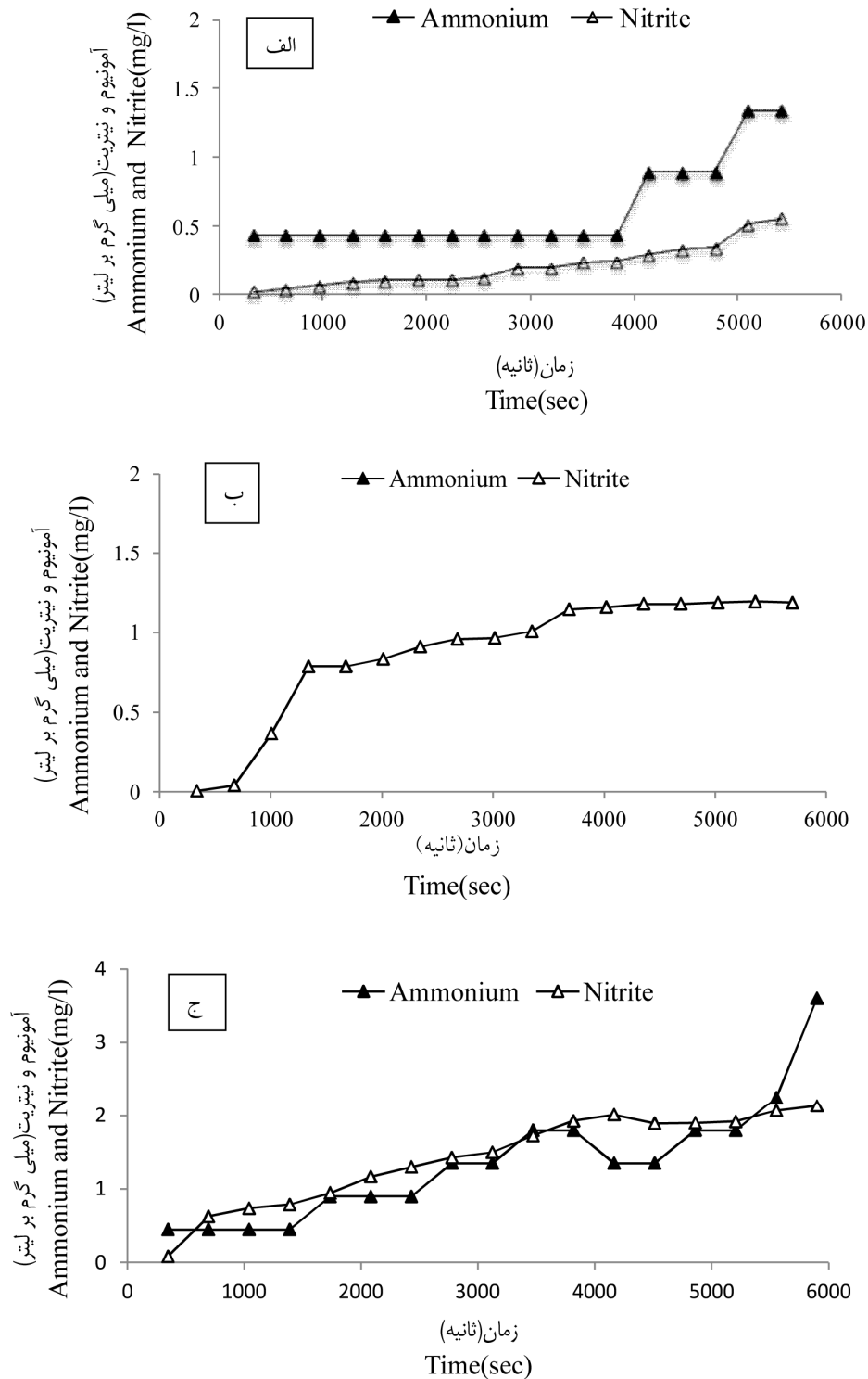
شکل 7- اثر غلظت نانوذرات بر مقادیر آمونیوم و نیتريت اندازه‌گیری شده در زه‌آب: (الف): 1 گرم بر لیتر، (ب): 2 گرم بر لیتر و (ج): 3 گرم بر لیتر (غلظت نیتريت 150 میلی‌گرم بر لیتر، سرعت آب منفذی 0/16 میلی‌متر بر ثانیه).
