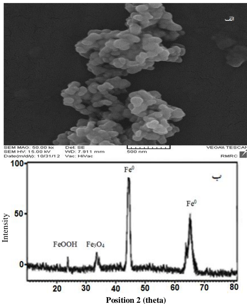
شکل 2- (الف): تصویر SEM نانوذرات آهن صفر ظرفیتی پایدار شده، (ب): دیاگرام XRD نانوذرات آهن صفر ظرفیتی پایدار شده با کربوکسی متیل سلولز.
