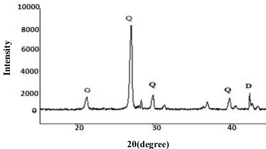
شکل 4- طیف XRD خاک شنی مورد مطالعه (D: دولومیت، Q: کوارتز و G: گئوتیت). Figure 4- XRD spectra of sand particle (D: Dolomite, Q: Quartz and G: Goethite).
