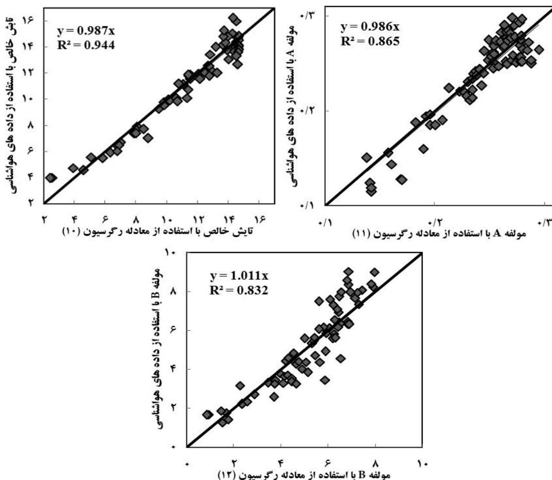
شکل ۲- پراکنش نتایج مؤلفه‌های R_n ، A و B حاصل از داده‌های هواشناسی و معادلات رگرسیونی
