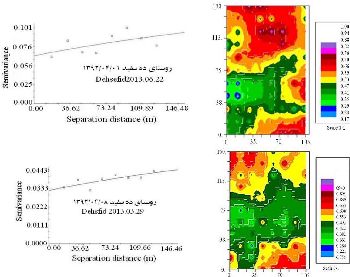
شکل ۴- نیم تغییرنما و نقشه کریجینگ غلاف‌های نخود آلوده به هلیوتیس در روستای ده سفید در سال ۱۳۹۲
