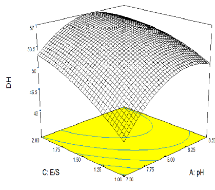
شکل ۲ نمودار سه بعدی اثر متغیرهای نسبت های آنزیم به سوبسترا و pH بر درجه هیدرولیز
