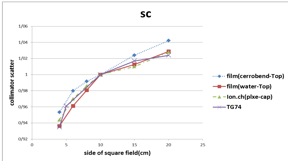
شکل ۴: فاکتورهای خروجی بدست آمده از اتاقک یونش، فیلم EBT2 با Top های آب و سروبند و مقادیر ارائه شده توسط AAPM در گزارش TG74.
