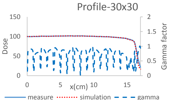
شکل ۵: منحنی های PDD و پروفایل انرژی 6 MV برای میدان های 4×4، 10×10 و 30×30 cm 2
