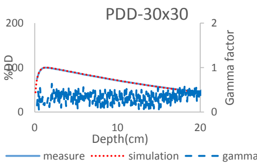
شکل ۵: منحنی های PDD و پروفایل انرژی 6 MV برای میدان های 4×4، 10×10 و 30×30 cm 2
