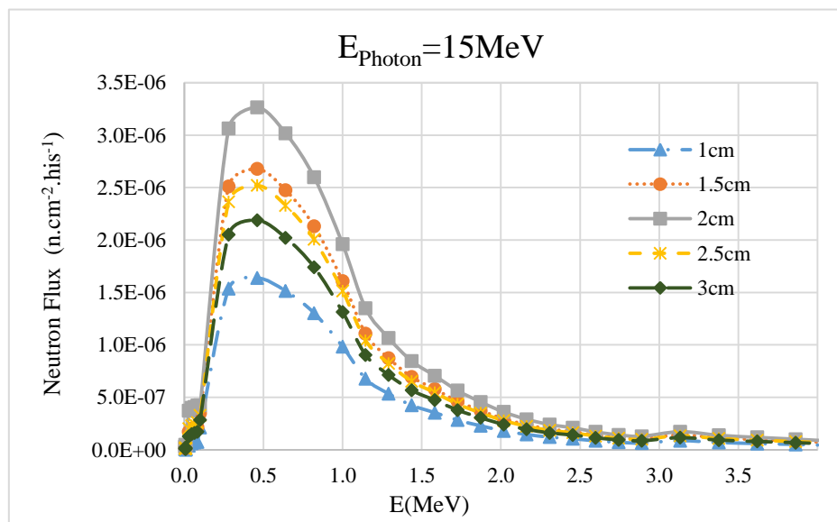
شکل ۳: شار نوترونی برای استوانه تنگستن با ضخامتهای مختلف و انرژی فوتون تابشی 15MeV
