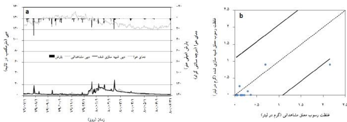
شکل ۶. مقایسه گرافیکی دبی مشاهده‌ای و شبیه‌سازی شده ۱۳۸۰-۱۳۷۹ در دوره اعتبارسنجی (a) و پلات پراکنش غلظت رسوب مشاهده‌ای و شبیه‌سازی شده در دوره اعتبارسنجی ۱۳۸۰-۱۳۷۸ در سطح اطمینان ۹۵ درصد (b)
