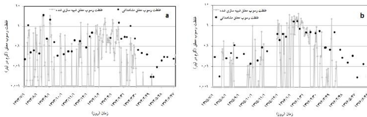
شکل ۴. مقایسه گرافیکی غلظت رسوب معلق مشاهداتی و شبیه‌سازی شده ۱۳۷۴-۱۳۷۶ (a) و ۱۳۷۵-۱۳۷۶ (b) در دوره واسنجی
