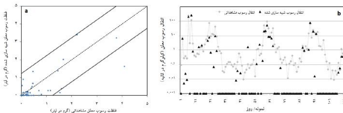
شکل ۵. نمودار پراکنش غلظت رسوب معلق مشاهده‌ای و شبیه‌سازی شده در دوره واسنجی (۱۳۷۶-۱۳۷۳) در سطح اطمینان ۹۵ درصد (a) و مقایسه گرافیکی ۱۱۱ نمونه انتقال رسوب معلق مشاهده‌ای و شبیه‌سازی شده در دوره واسنجی (b)
