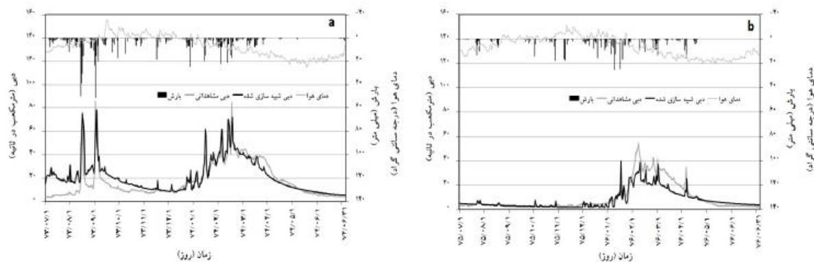
شکل ۲. مقایسه گرافیکی دبی مشاهداتی و شبیه‌سازی شده ۱۳۷۴-۱۳۷۶ (a) و ۱۳۷۵-۱۳۷۶ (b) در دوره واسنجی
