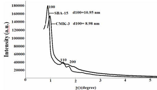
سویز شماره ۱: الگوی پراش پرتو ایکس نانوحفره سیلیسی SBA-15 و نانوحفره کربنی CMK-3
