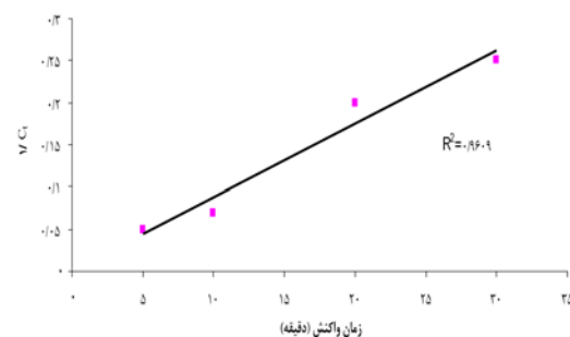
نمودار شماره ۶: سینتیک حذف فورفورال
