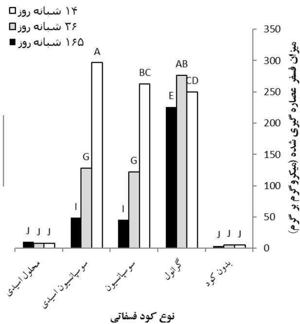
نمودار ۱- میزان فسفر قابل جذب در خاک خوشنام در طول زمان، پس از افزودن اشکال مختلف کود حاوی فسفات
