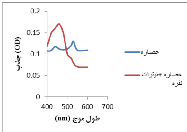
شکل ۲- طیف جذبی از دستگاه اسپکتروسکوپی نانوذرات نقره تولید شده توسط آلوئه ورا
