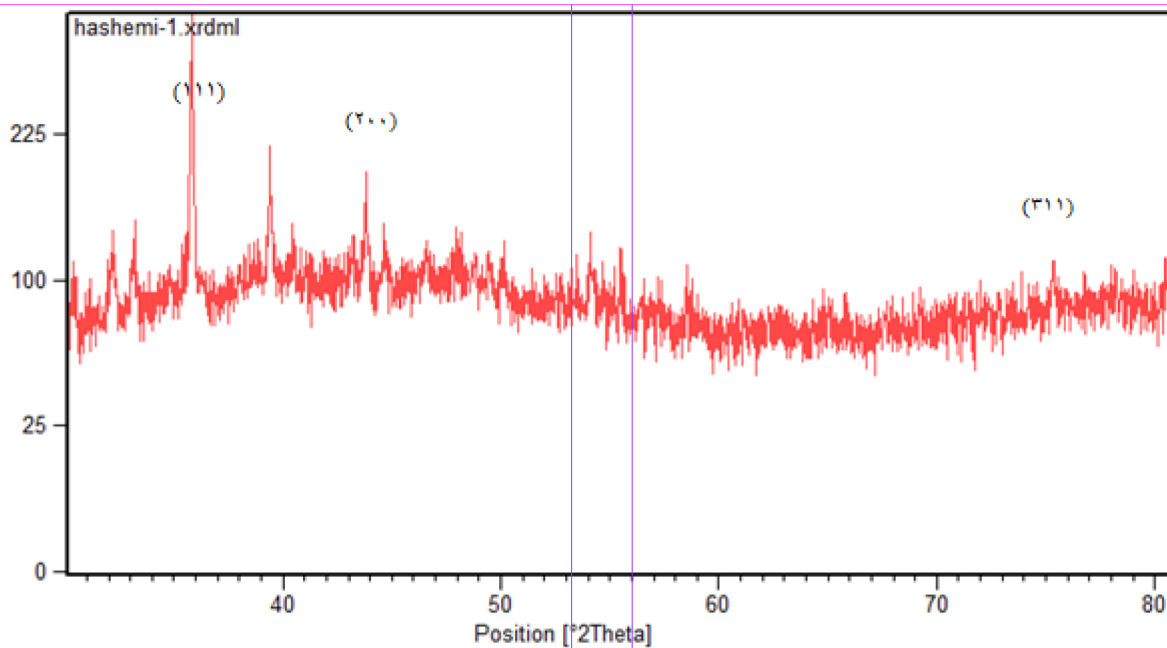
شکل ۳- پراش پودری پرتو ایکس (XRD) نانوذرات نقره سنتز شده توسط آلوتهورا
