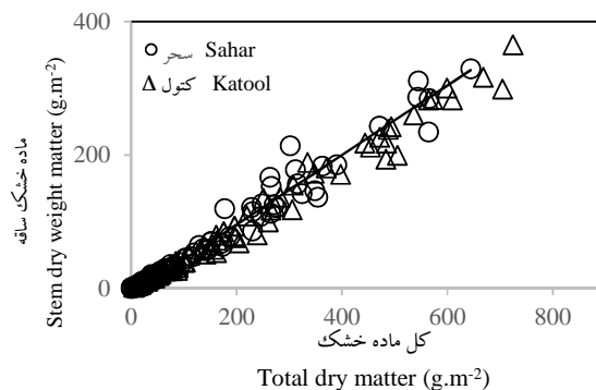
شکل ۴- رابطه بین وزن خشک تجمعی ساقه و وزن خشک کل بوته از کاشت تا مرحله R 5 در ارقام سحر و کتول سویا Fig. 4. Relationship between cumulative stem dry weight and total dry matter (planting to R 5 growth stage) in
