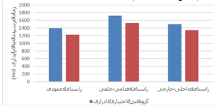
نمودار ۱. مقایسه زمان رسیدن به پایدار بودن در سه راستا بین زنان با و بدون بی‌اختیاری اداری
