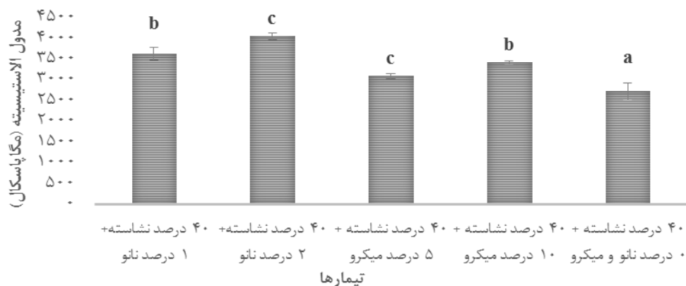
شکل ۴. تأثیر نانو و میکروالیاف سلولزی بر مدول الاستیسیته نمونه‌های ساخته‌شده با ۴۰ درصد نشاسته (حروف لاتین متفاوت روی ستون‌ها نشان‌دهنده گروه‌بندی دانکن و وجود اختلاف معنی‌دار بین تیمارهاست)
