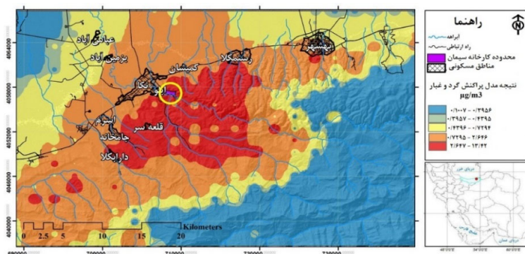
شکل ۳. نتیجه مدل‌سازی انتشار ذرات معلق در هوا با قطر 10 میکرون ( PM_{10} )
