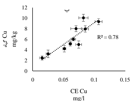
شکل 3- رابطه بین میزان Cu اندازه‌گیری شده توسط الف) عصاره‌گیر DTPA در خاک و ب) DGT (C E ) در خاک با مقادیر اندازه‌گیری شده در گیاه
