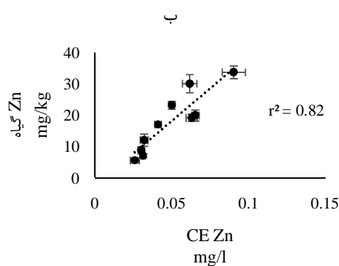
شکل 2- رابطه بین میزان Zn اندازه‌گیری شده توسط الف) عصاره‌گیر DTPA در خاک و ب) DGT (C E ) در خاک با مقادیر اندازه‌گیری شده در گیاه
