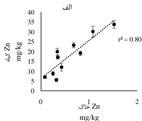
شکل 2- رابطه بین میزان Zn اندازه‌گیری شده توسط الف) عصاره‌گیر DTPA در خاک و ب) DGT (C E ) در خاک با مقادیر اندازه‌گیری شده در گیاه
