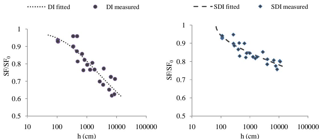
شکل 4- تغییرات SF/SF_0 به صورت تابعی از مکش ماتریک خاک ( h ) در دو سامانه آبیاری
