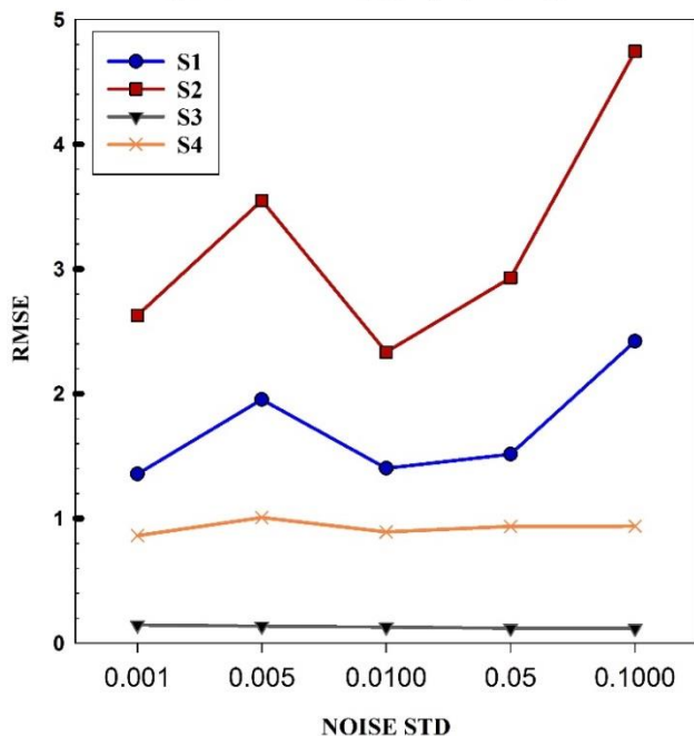
شکل ۷- اثر تغییر خطای اندازه گیری مرز باز
