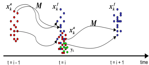
شکل ۱: اجرای طرح همگونسازی داده‌ها با فیلتر گروهی کالمن [۱]
