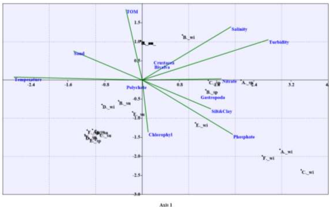
شکل ۹: نتایج آزمون ارتباط کانونی برای متغیرهای محیطی و گروه‌های غالب ماکروبتوتوزی در ایستگاه‌های نمونه‌برداری (حروف A, B, C, D, E, F به ترتیب نشان‌دهنده ترانسکت‌های بساتین، شاهد، پل ولایت، حاشیه خلیج، بیدخون و پتروشیمی و حروف اختصاری sp, su, wi و au به ترتیب نشان‌دهنده فصول بهار، تابستان، پاییز و زمستان است).
