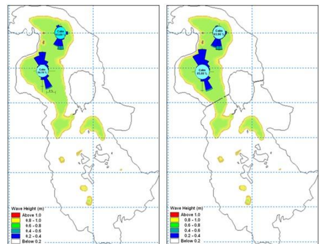
شکل ۹: گل‌موج حاصل از شبیه‌سازی‌ها در نقاط مختلف دریاچه در حالت کم‌آبی و برای حالت با و بدون میان‌گذر
