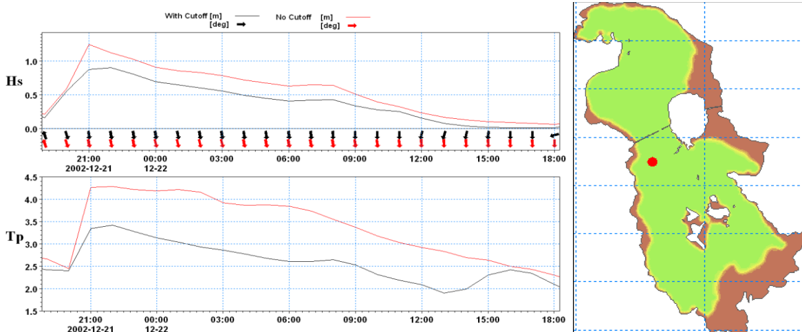
شکل ۷: مقایسه سری زمانی امواج برای دو حالت وجود و عدم وجود میان‌گذر در نقطه‌ای در جنوب میان‌گذر دریاچه
