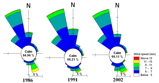
شکل ۸: مقایسه گلباد حاصل از میدان باد WRF را در سه سال مختلف و برای یک نقطه در میان دریاچه
