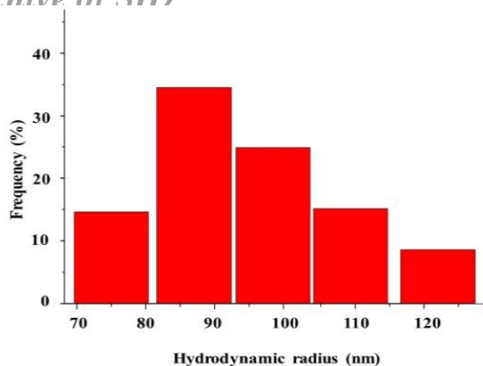
نمودار شماره ۱: نمودار پراکندگی نور دینامیکی (DLS) نانوذرات اکسید نیکل در آب دوبار تقطیر
