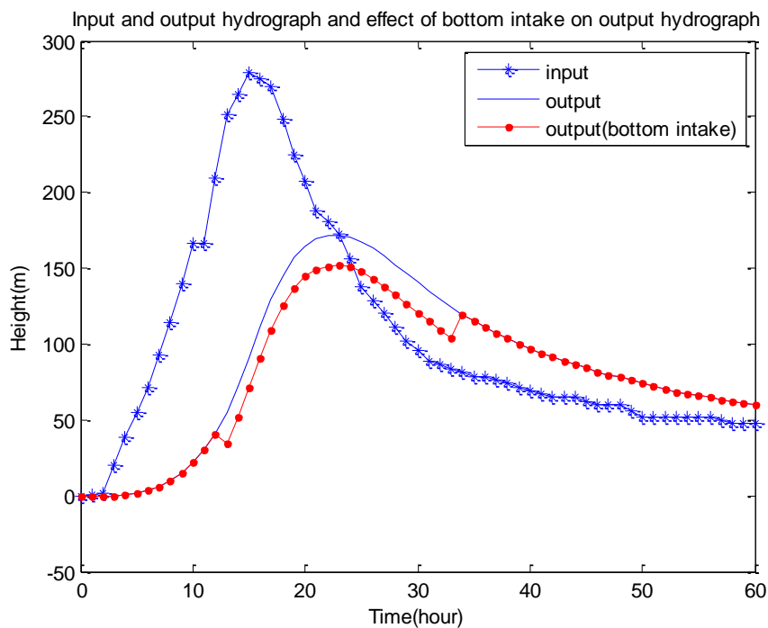
Fig. 9- Effect of lower gate opening or bottom intake on output hydrograph شکل ۹- اثر باز شدن دریچه تحتانی با آبگیر بر هیدروگراف خروجی
