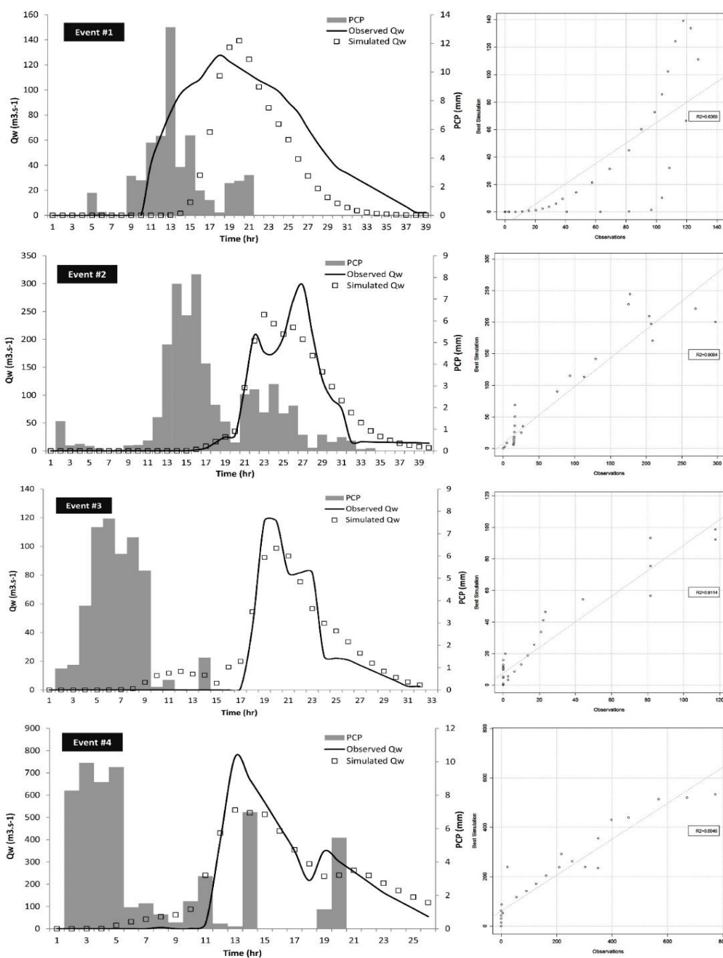
شکل ۳- دبی شبیه‌سازی شده (Simulated Qw) در برابر دبی مشاهده‌ای (Observed Qw) همراه با هیئوگراف بارش (PCP) بر اساس وقایع مختلف رگباری
