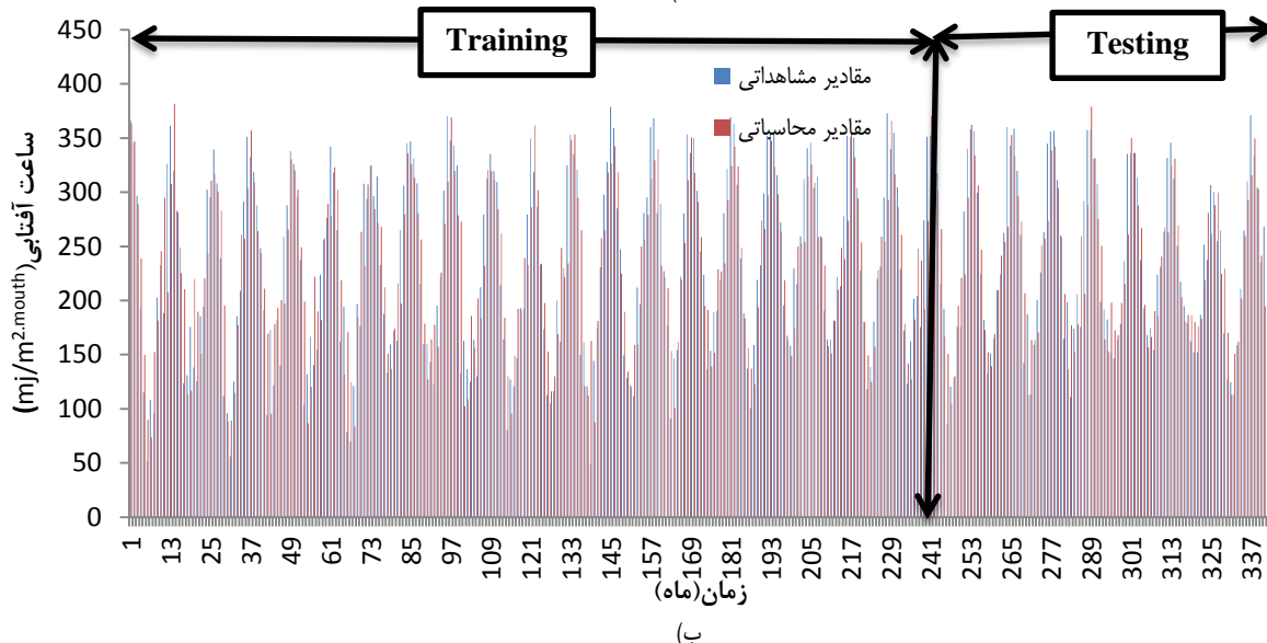
شکل ۹- الف و ب)- مقادیر مشاهده‌ای و پیش‌بینی شده ساعات آفتابی ایستگاه سینوپتیک تبریز با شبکه بیزین و رگرسیون خطی چندمتغیره (ترکیب ۳) بخش آموزش و صحت سنجی
