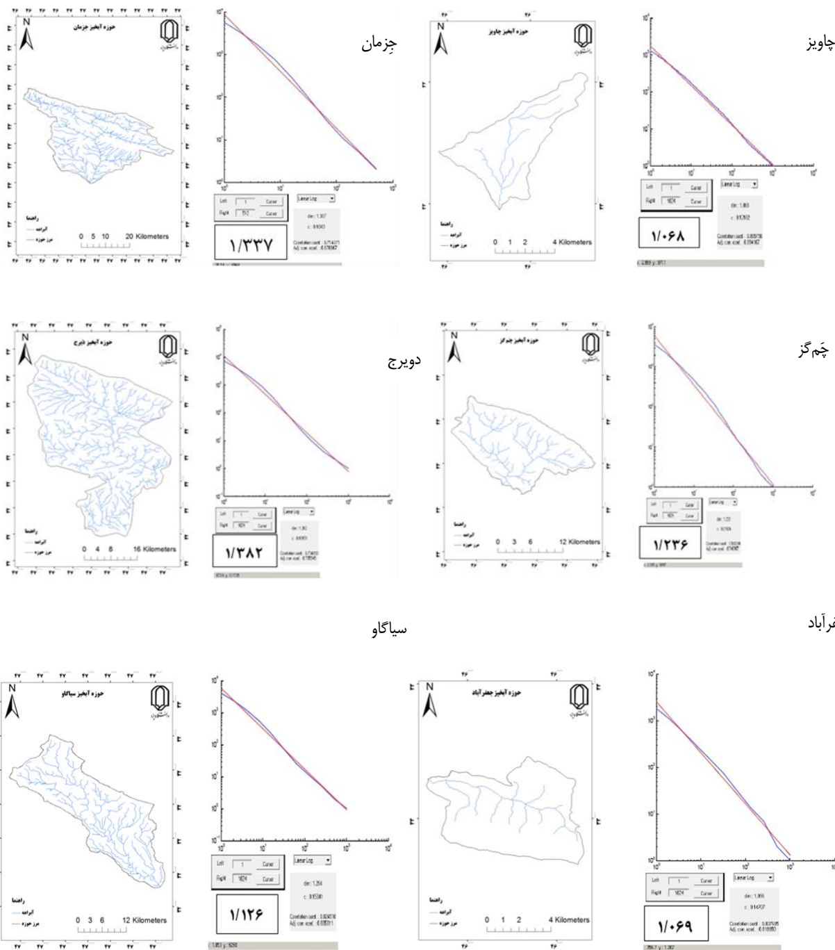
ادامه شکل ۲- شبکه هیدروگرافی و بعد فراکتال حوزه‌های آبخیز قبل از اصلاح شبکه هیدروگرافی Continued Figure 2. Hydrographic network and fractal dimension of watersheds before hydrographic network modification
