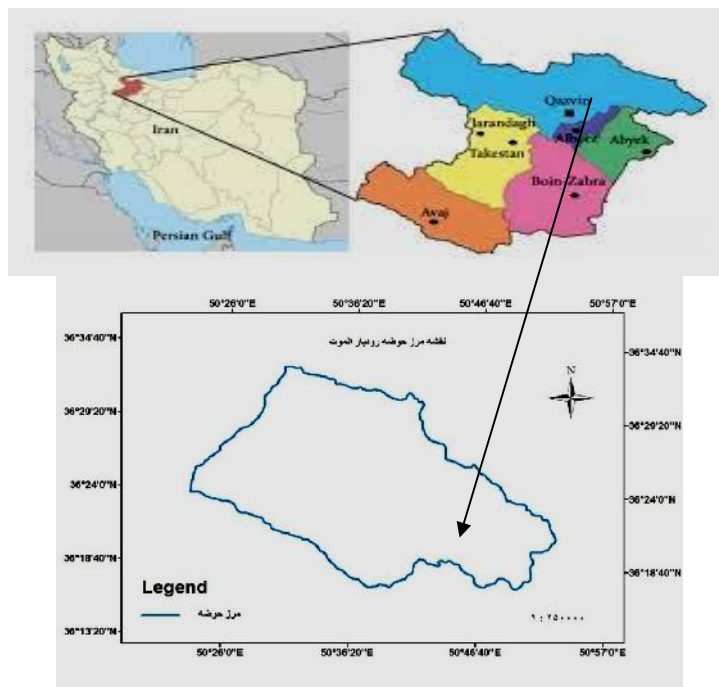
شکل ۱- موقعیت حوزه آبخیز رودبار الموت در استان قزوین Figure 1. Position of the Roudbar Alamut Basin in Qazvin province and Iran
