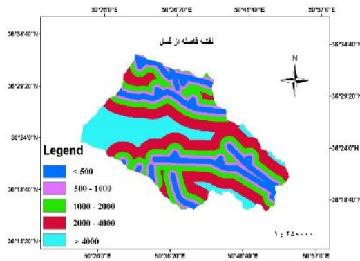
شکل ۸- نقشه فاصله از گسل حوزه آبخیز الموت Figure 8. Alamoort watershed distance from fault map
