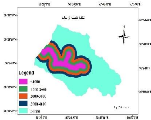
شکل ۵- نقشه فاصله از جاده حوزه آبخیز الموت Figure 5. Alamoot watershed distance from road map
