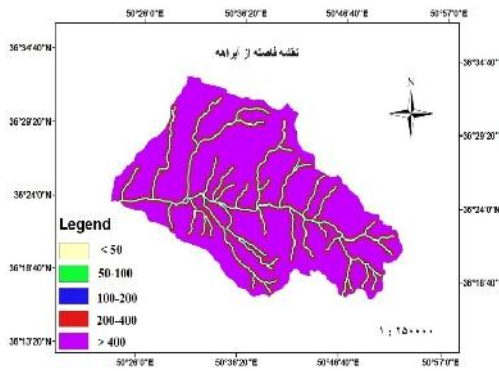
شکل ۷- نقشه فاصله از آبراهه حوزه آبخیز الموت Figure 7. Alamoort watershed distance from river map
