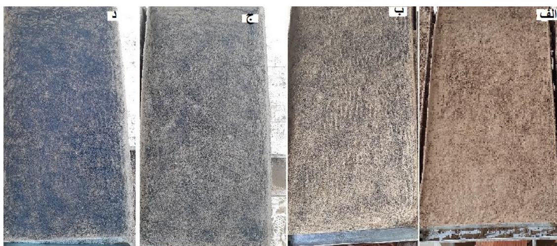
شکل ۲- نمایی از کرت‌ها با مقادیر مختلف زغال‌زیستی صفر (شاهد) (الف)، ۰/۴ (ب)، ۰/۸ (ج) و ۱/۶ (د) تن بر هکتار Figure 2. A view from plots with different amounts of biochar 0 (control) (a), 0.4 (b), 0.8 (c) and 1.6 (d) t ha -1
