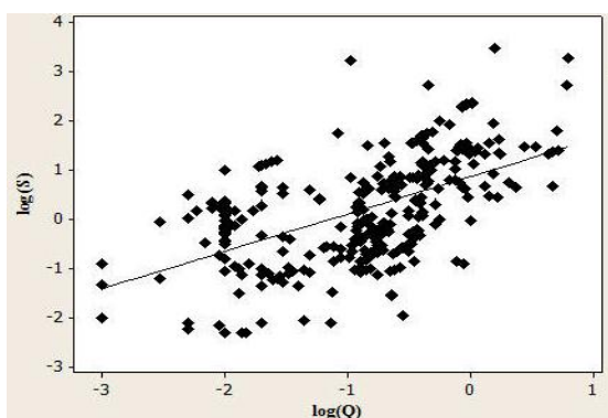
شکل ۴- نمودار خطی بر اساس لگاریتم دبی جریان و رسوب معلق در ایستگاه مرویل ( R^2=0.32 ) Figure 4. Linear graph, based on the logarithm of the flow discharge and the suspended sediment in the Marvil station ( R^2=0.32 )
