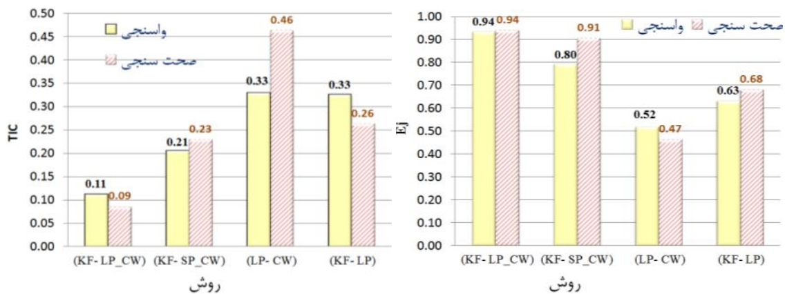
شکل ۷- نمودار متوسط معیار ارزیابی Eij و TIC در مرحله واسنجی و صحت‌سنجی Figure 7. The average value of Eij and TIC for calibration and test step
