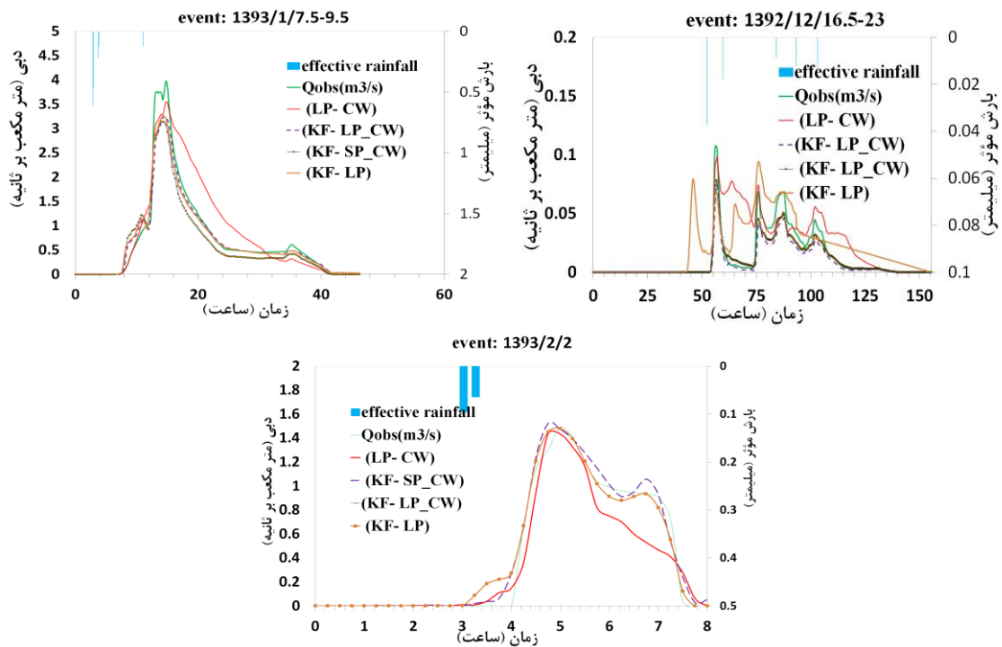
شکل ۵- شبیه‌سازی روش‌های مورد مطالعه در حوضه لیتقوان در مرحله صحت‌سنجی Figure 5. The simulation of studied methods in Lighvan basin for test step
