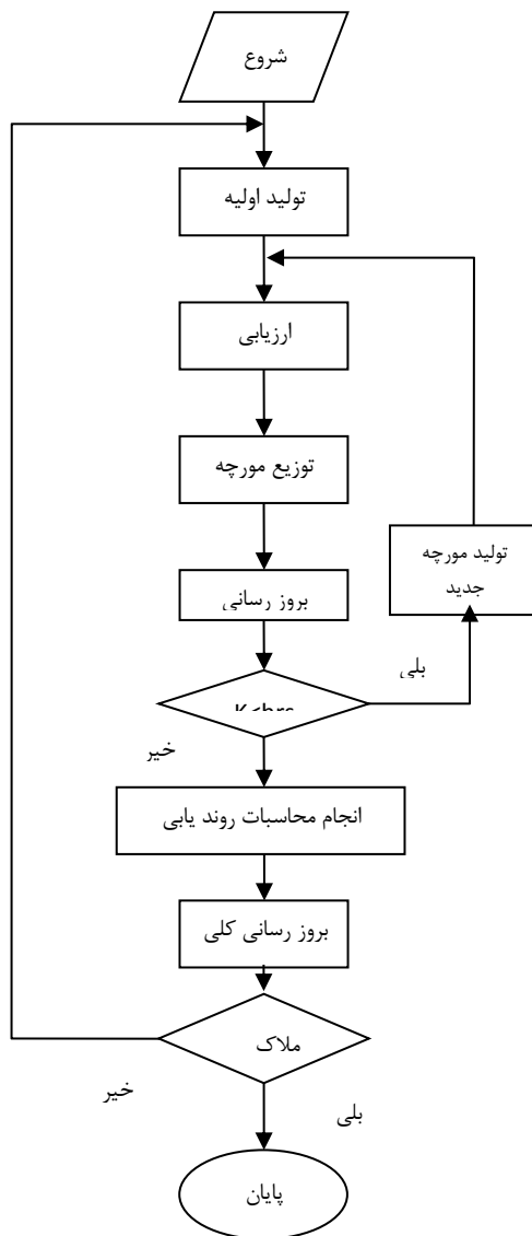
شکل ۴- نمودار گردش روشی مدل شبیه سازی و بهینه سازی Figure 4. The flowchart of simulation and optimization model
