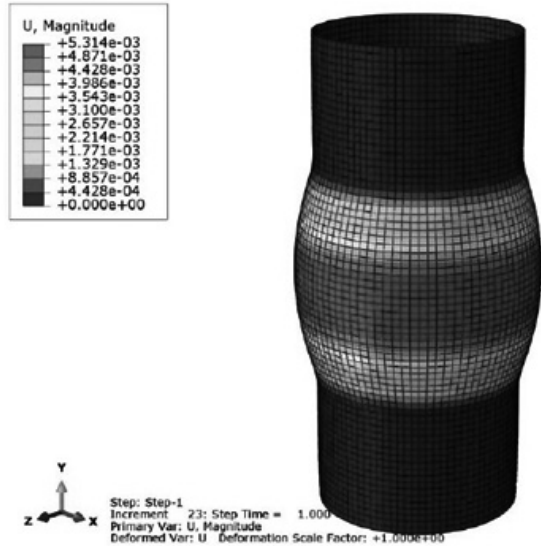
شکل ۹- لوله‌ی شبیه‌سازی شده در نرم‌افزار آباکوس تحت فشار ۲۰ MPa
