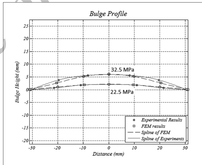
شکل ۱۰- اسپ‌پی لاین عبور داده شده از نقاط برداشت شده از روی پروفیل لوله در آزمایش و شبیه‌سازی برای فشارهای ۲۲/۵ MPa و ۳۲/۵ MPa
