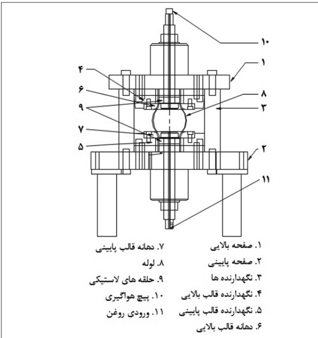
شکل ۴- دستگاه آزمایش بادکردگی آزاد لوله
