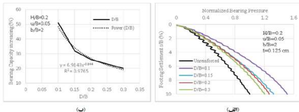
شکل شماره (۵): نتایج مربوط به قطر بازشو لایه ژئوسل (غفارپور و شیبانی، ۱۳۹۳)
