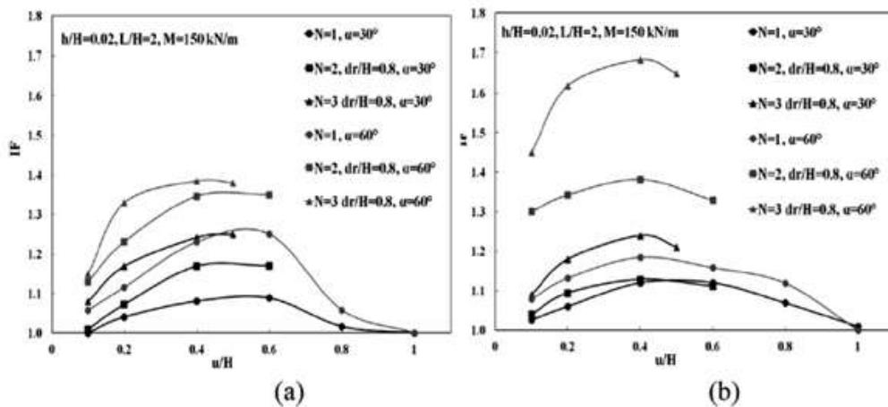
شکل شماره (۱۴): تأثیر تعداد لایه مسلح کننده در پایداری شیروانی (a) برای خاک ماسه‌ای و (b) برای خاک رسی در پژوهش مهدی پور و همکاران (۲۰۱۳)
